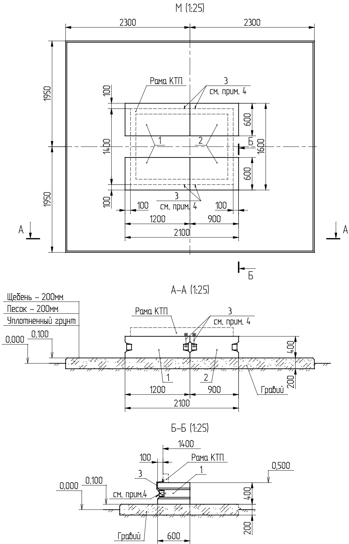
Рис. 5 КТПТАС - В/К - 400/10/0,4 кВА
