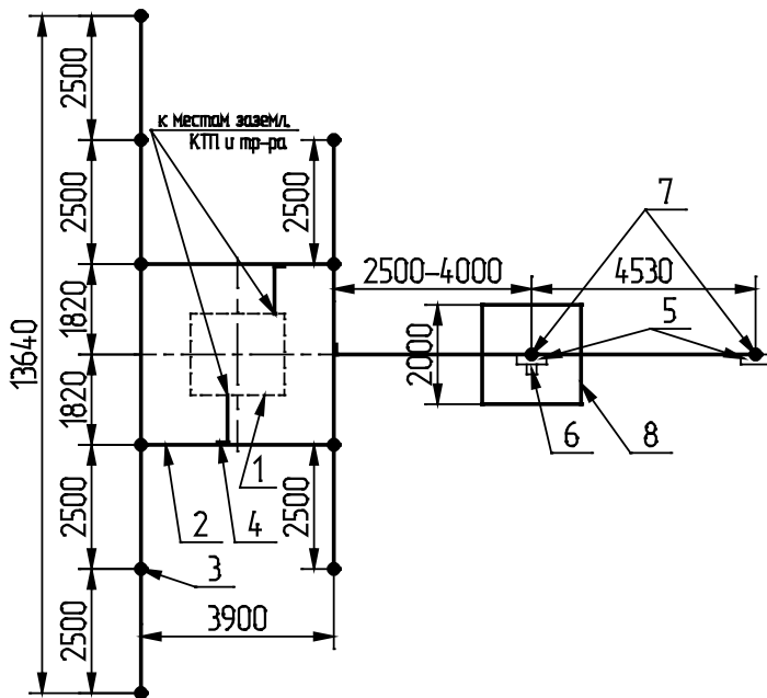
Рис. 3 КТПТАС – В/К – 400/10/0,4 кВА
