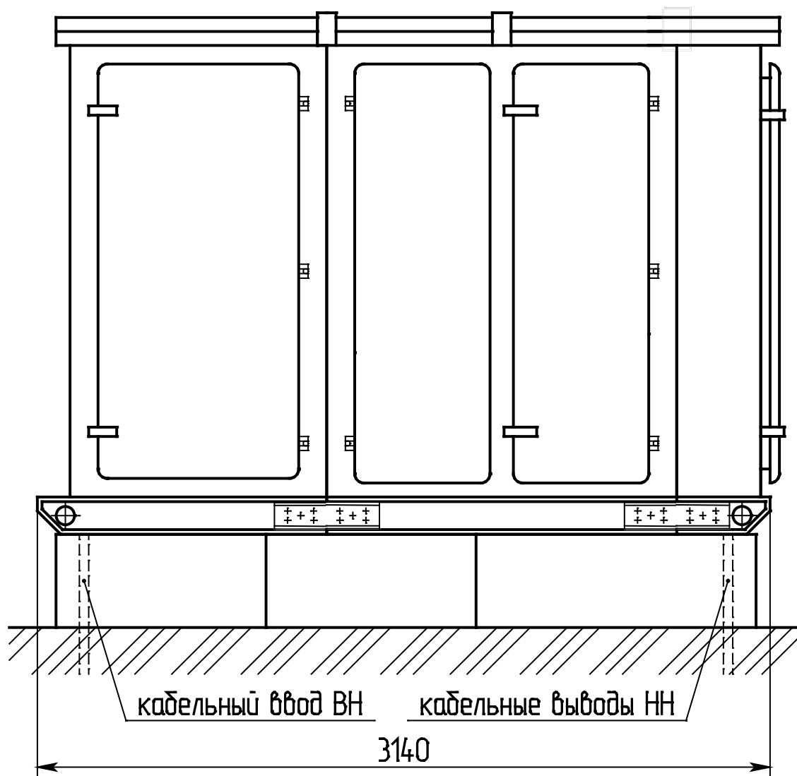
Рис. 2 КТПТАС – К/К – 400/10/0,4 кВА
