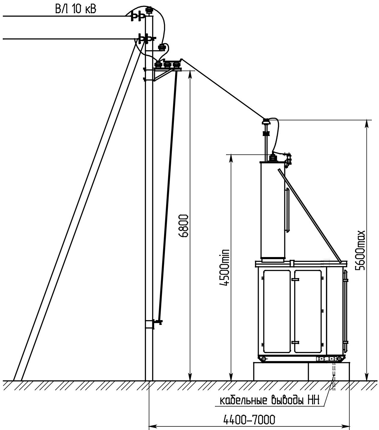
Рис. 1 КТПТАС – В/К – 400/10/0,4 кВА
