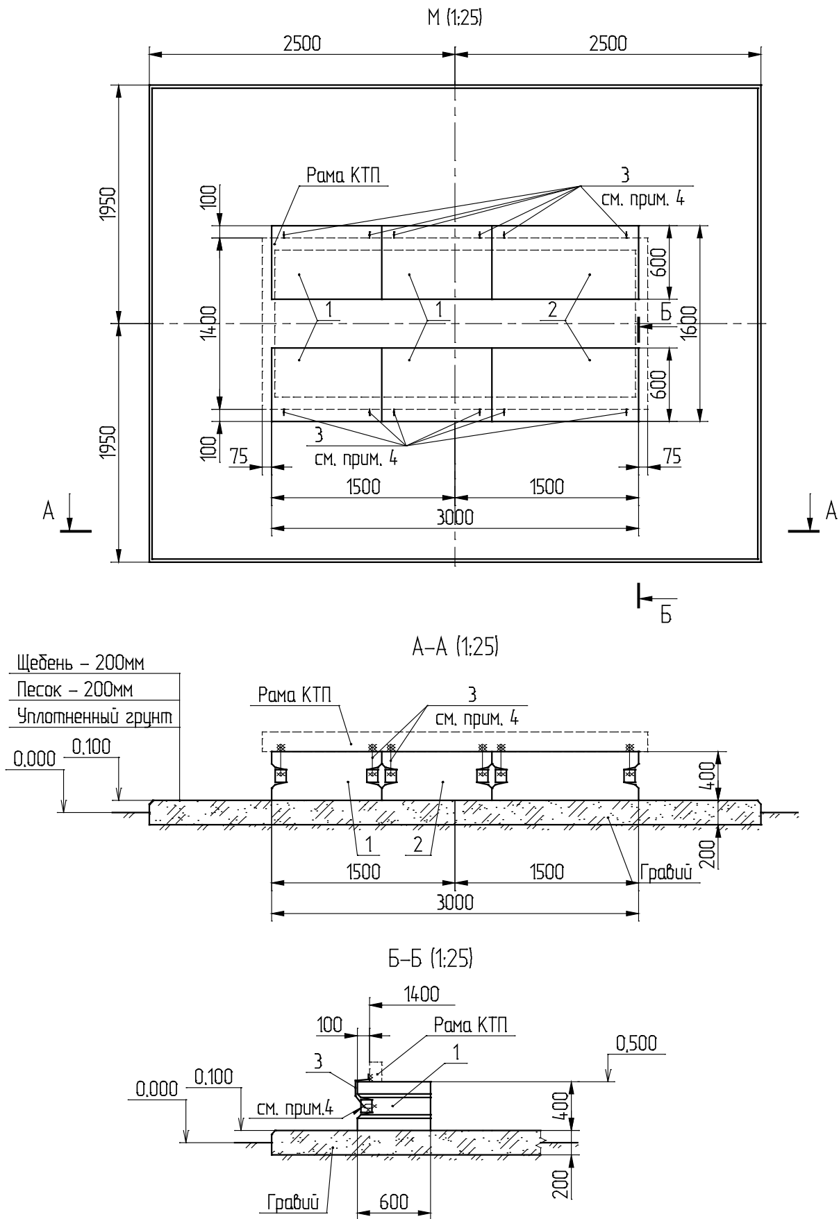
Рис. 6 КТПАС – К/К – 400/10/0,4 кВА
