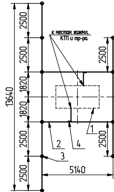
Рис. 4 КТПТАС – К/К – 400/10/0,4 кВА
